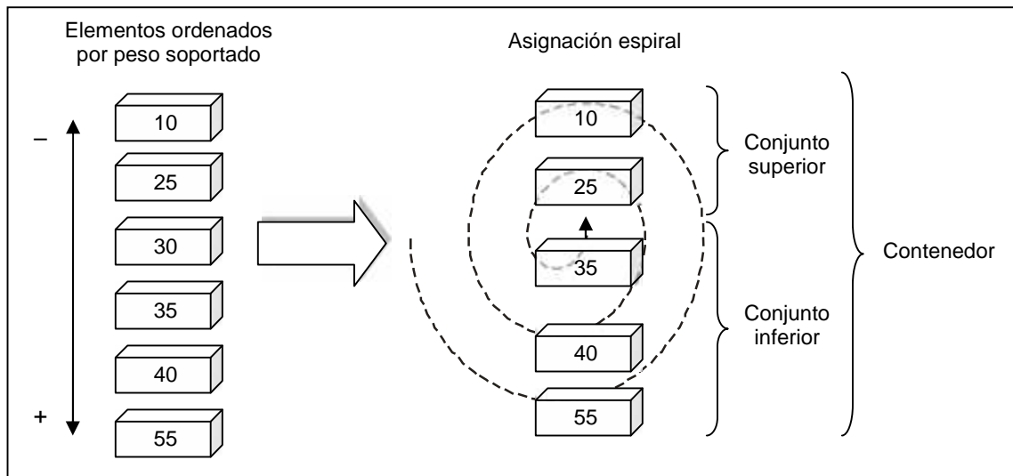
Figura 5.14. Asignación espiral.
