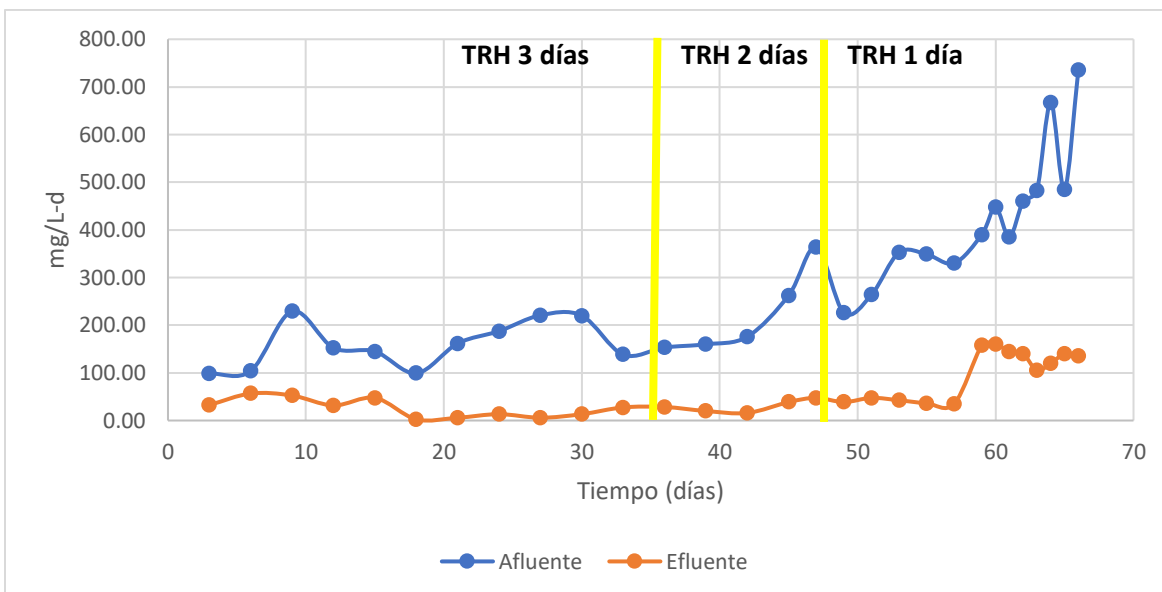
Figura 3.2. Perfiles de carga y descarga de la DQO en el afluente y efluente del tren de tratamiento 1.
