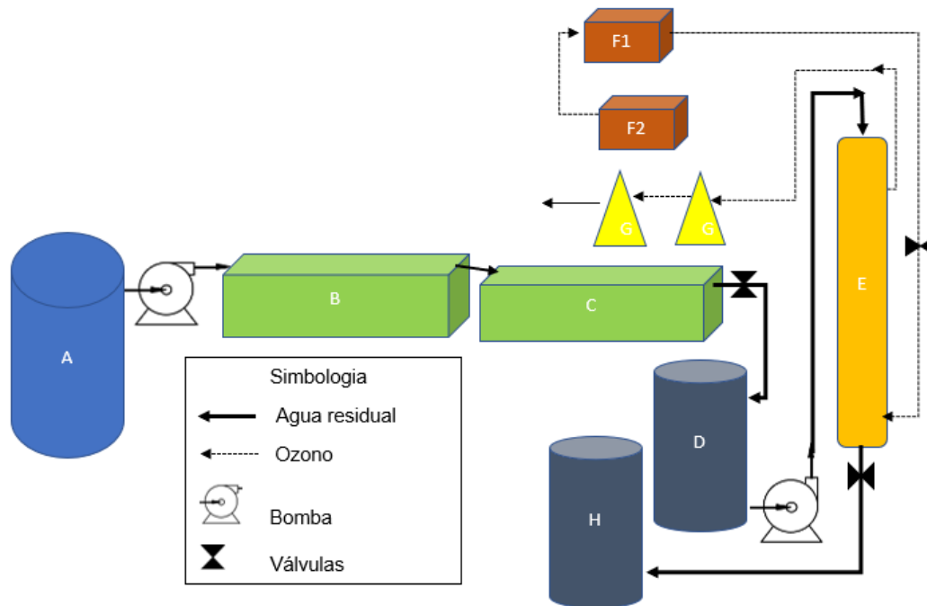
Figura 2.12. Diseño experimental, donde “A” es el depósito de agua residual, “B” humedal subsuperficial, “C” humedal superficial, “D” efluente del sistema de fitodepuración, “E” reactor O 3 /UV, “F1” generador de O 3 , “F2” compresor, “G” trampas de KI y “H” efluente final del tren de tratamiento.
