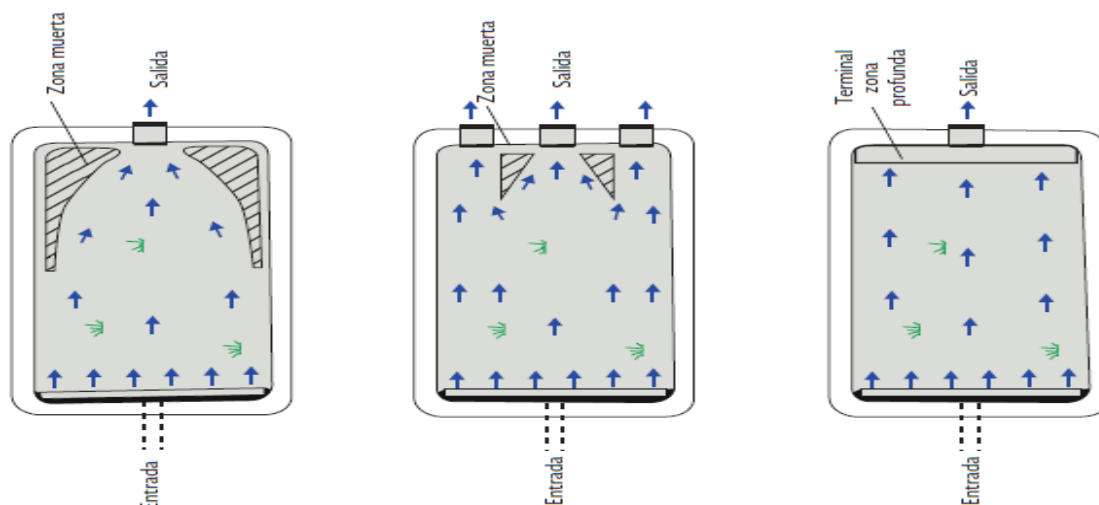
Figura 1.3. Efecto de las estructuras de entrada y salida en la distribución del flujo del agua en los humedales artificiales.
