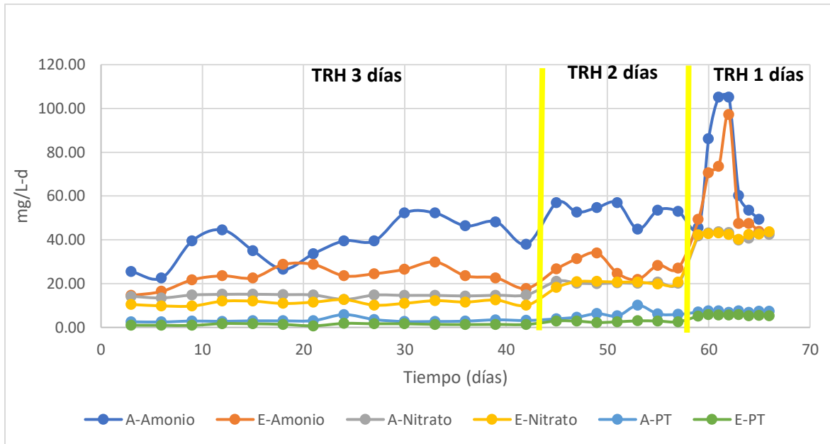
Figura 3.3. Perfiles de carga y descarga de amonio, nitrato y PT en el afluente y efluente del tren de tratamiento 1.
