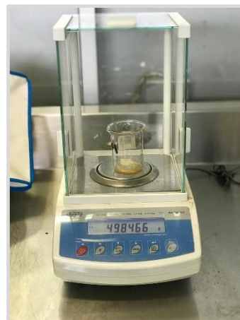
Figura 30 Pesado de grasa extraída en Balanza RADWAG AS 220/c.
